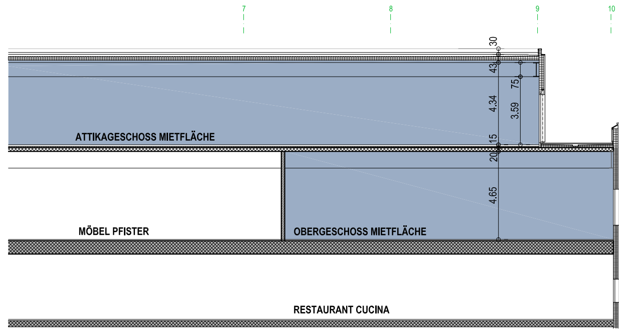
SCHNITT A-A
